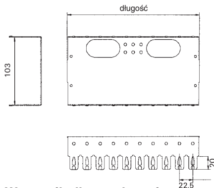
Wspornik dla przełącznic głównych
