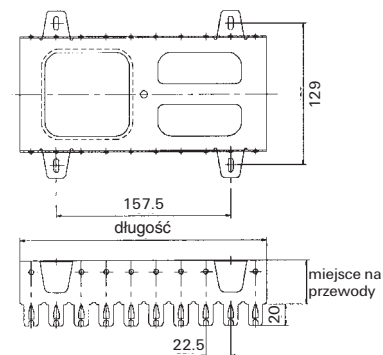
Wspornik dla szafek kablowych
