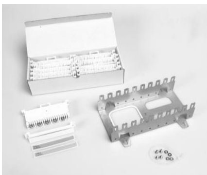
Blok łączówkowy do szafek kablowych
